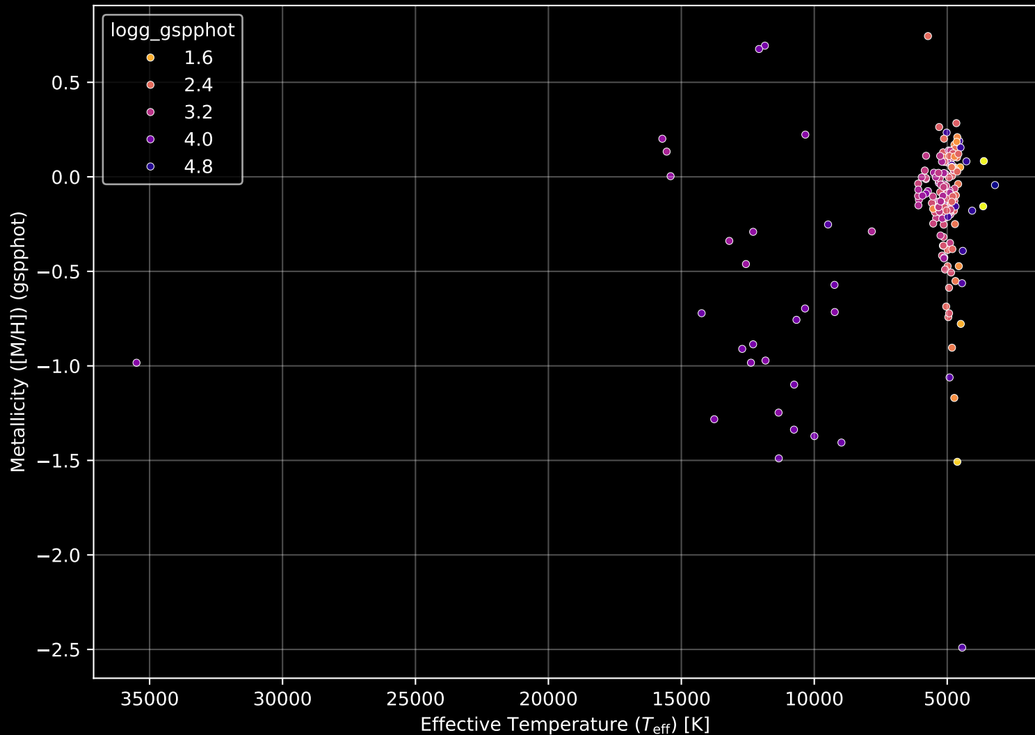
APOGEE DR17 Field: [199-04] Stellar Population Parameters (n= 202)
